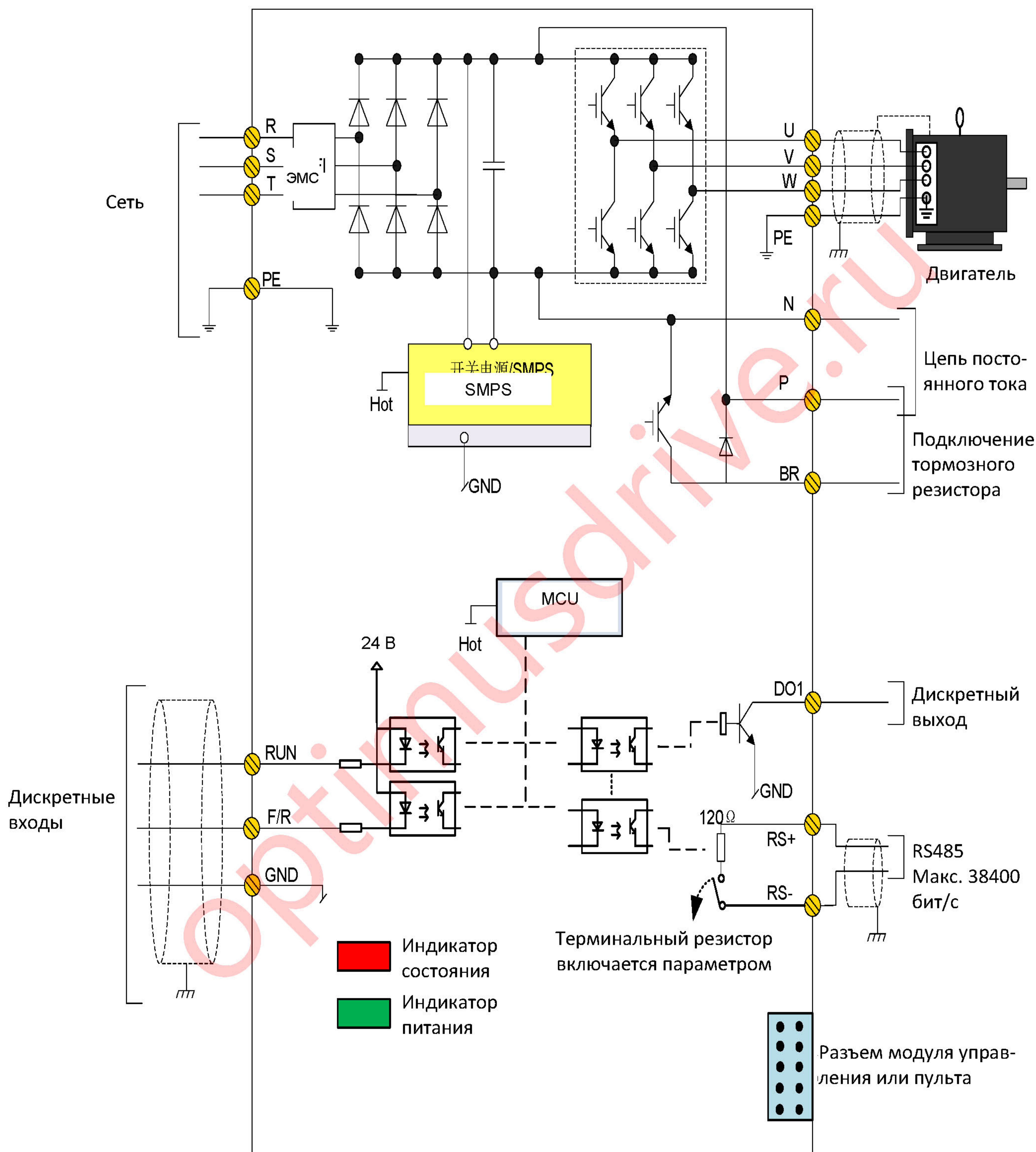
Силовой модуль PU01 (0.37-7.5 кВт)
