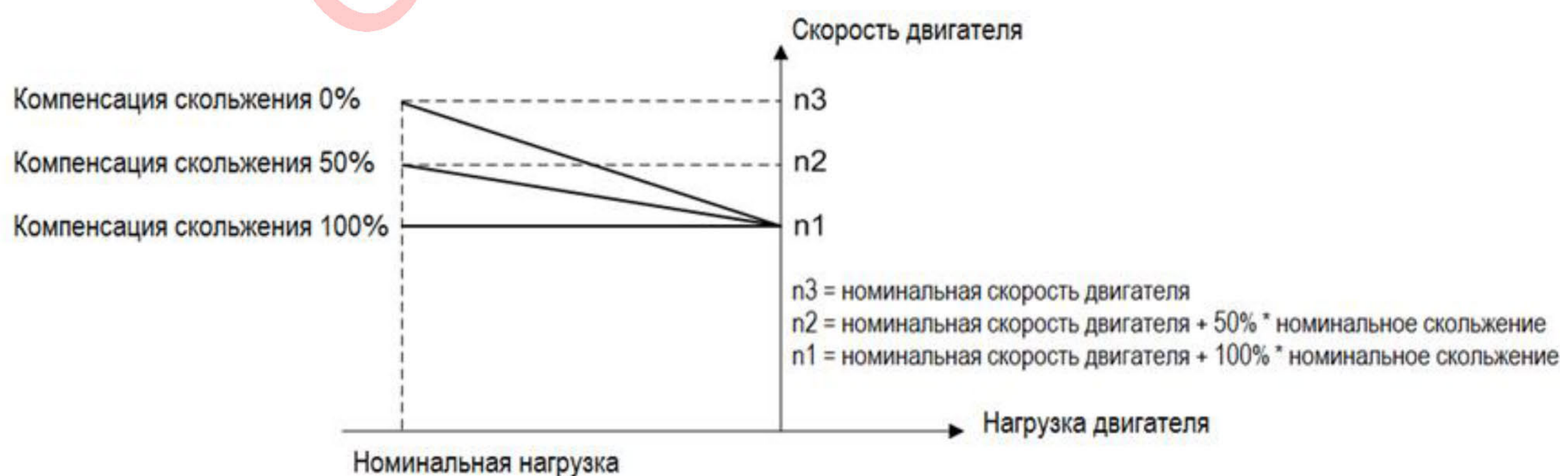
Компенсация скольжения в генераторном режиме
